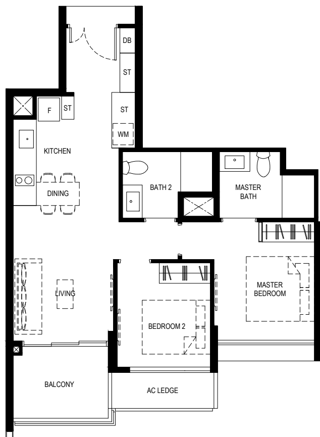
2BR-Pa
